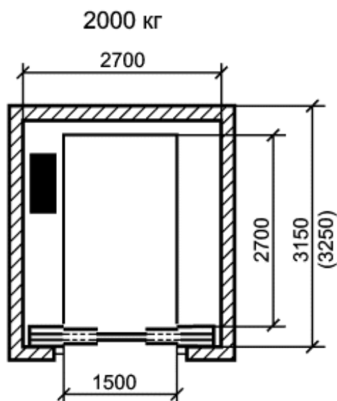
Высота кабины 2100. Высота дверного проема 2100
