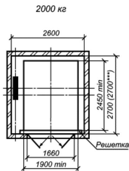
Высота кабины 2200. Высота дверного проема 2200
