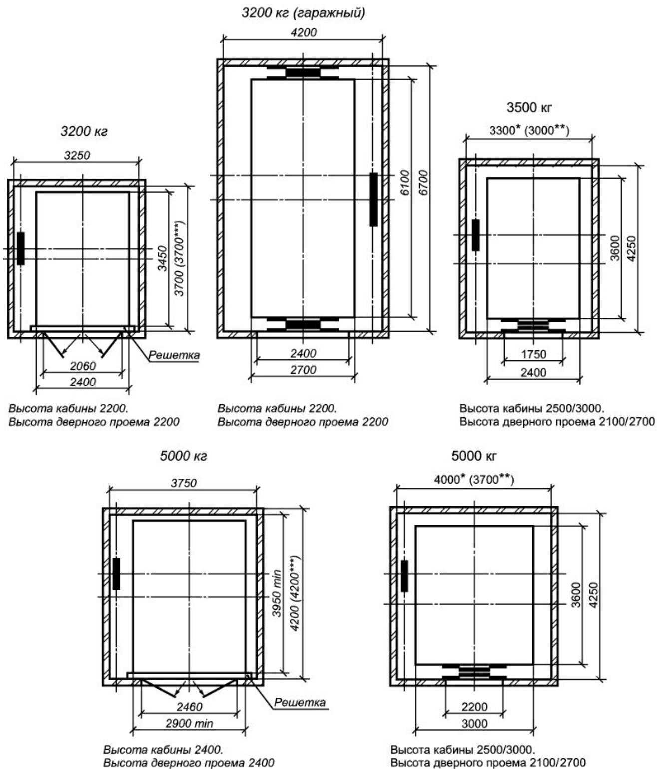
Рисунок 6 - Грузовые лифты категории В с дверями типов З и Р, лист 1
