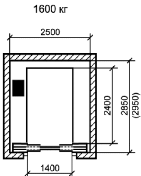
Высота кабины 2100. Высота дверного проема 2100
