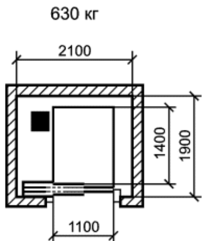
Высота кабины 2100. Высота дверного проема 2100
