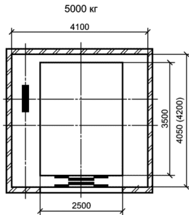
Высота кабины 2500. Высота дверного проема 2500
