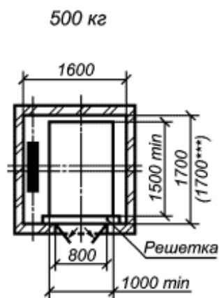
Высота кабины 2000. Высота дверного проема 2000
