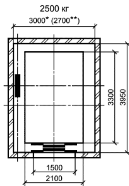
Высота кабины 2500/3000. Высота дверного проема 2100/2700
