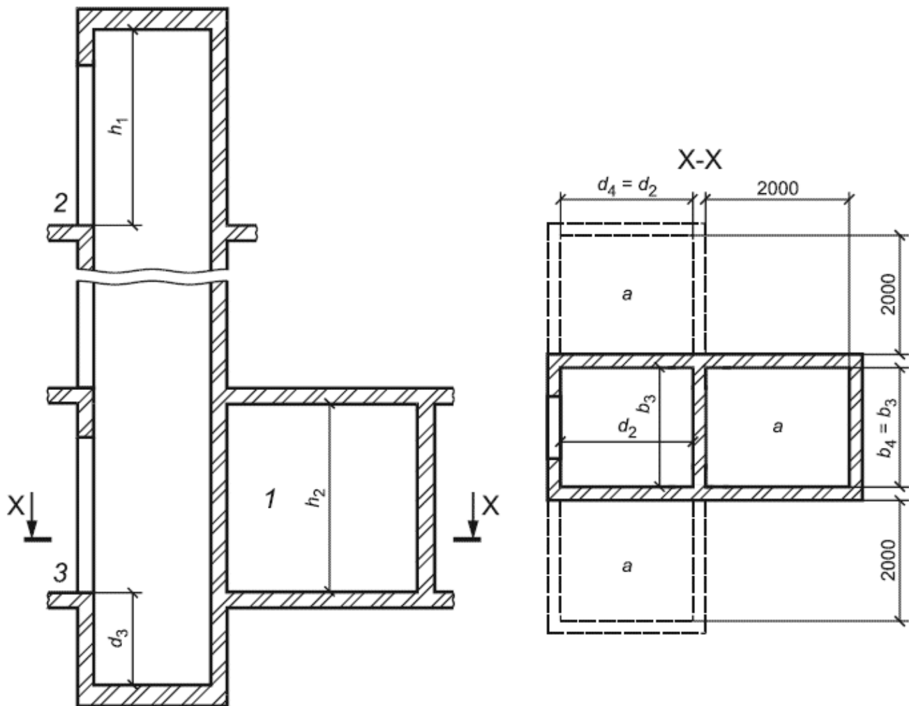
Рисунок 3 - Гидравлические грузовые лифты. Обозначения размеров шахты и машинного помещения
