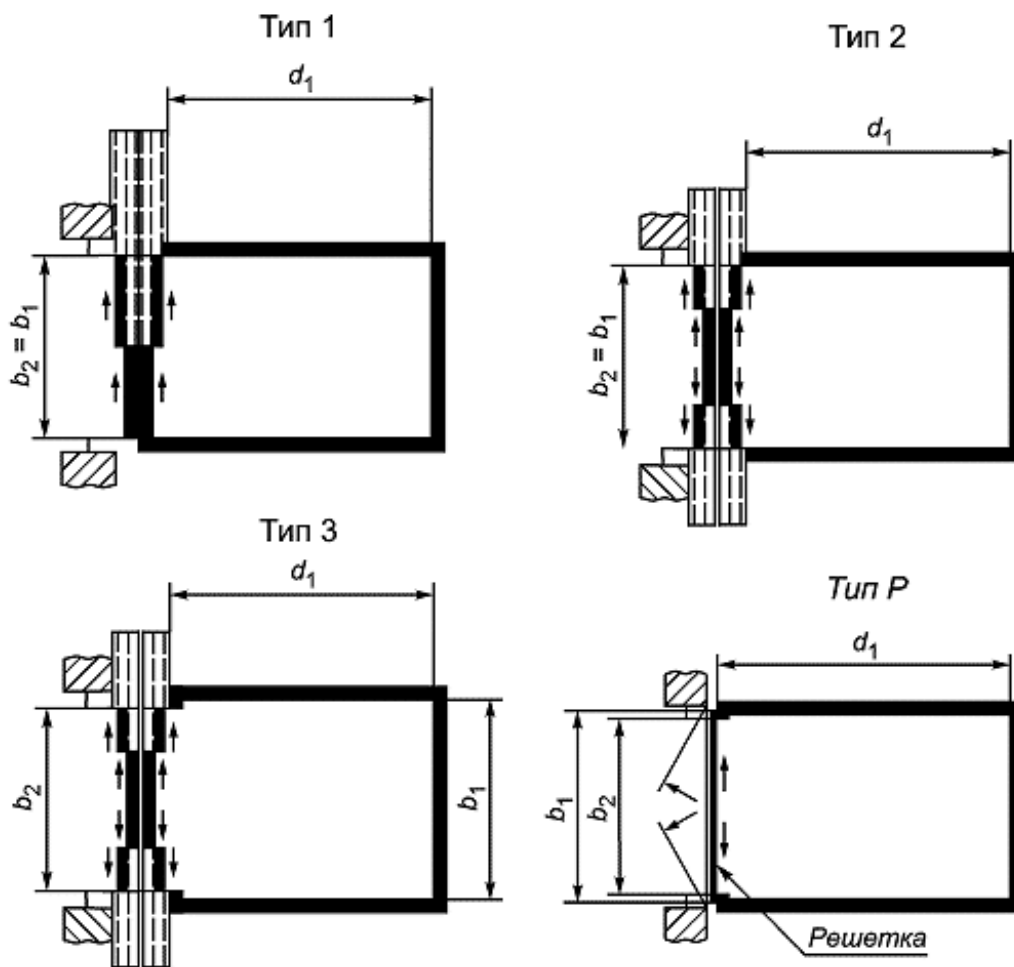
Двери шахты и кабины
