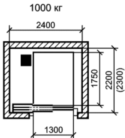
Высота кабины 2100. Высота дверного проема 2100
