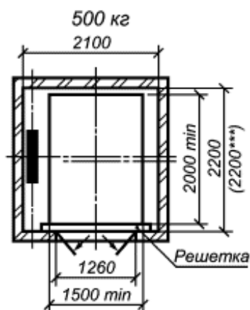
Высота кабины 2000. Высота дверного проема 2000
