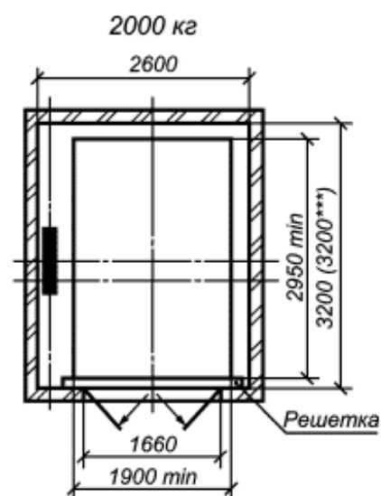
Высота кабины 2200. Высота дверного проема 2200
