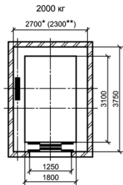
Высота кабины 2500/3000. Высота дверного проема 2100/2700
