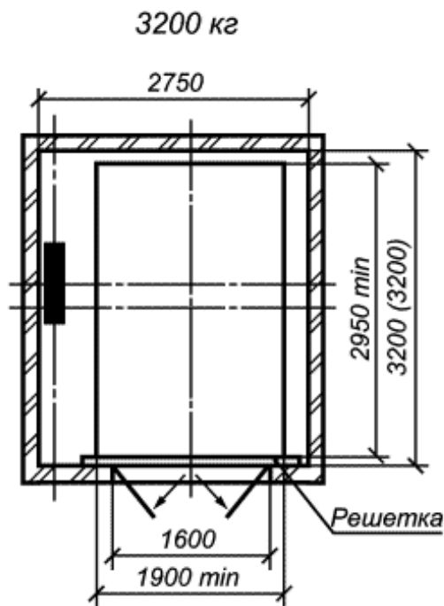
Высота кабины 2200. Высота дверного проема 2200
