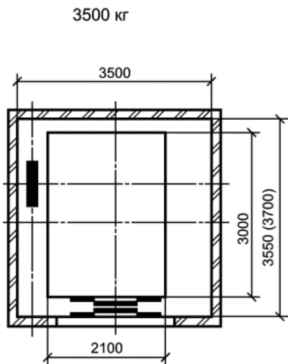
Высота кабины 2500. Высота дверного проема 2500
