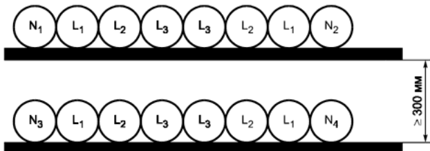
Рисунок Н.52.8 - Специальная конфигурация для 12 параллельных одножильных кабелей один выше другого (см. 523.7)
